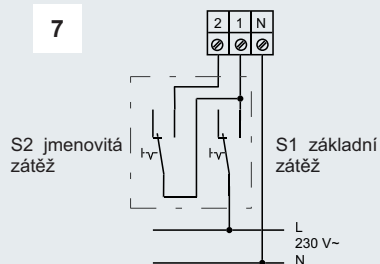
V-II 30/60, 30/100, možnost spínání základní zátěže
